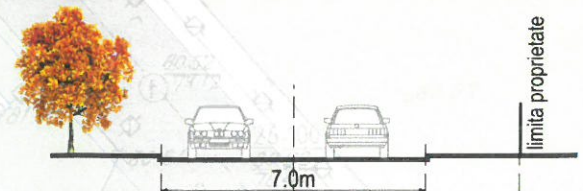
Profil B-B - str. Magnoliei - categoria a III-a, sc. 1:200
