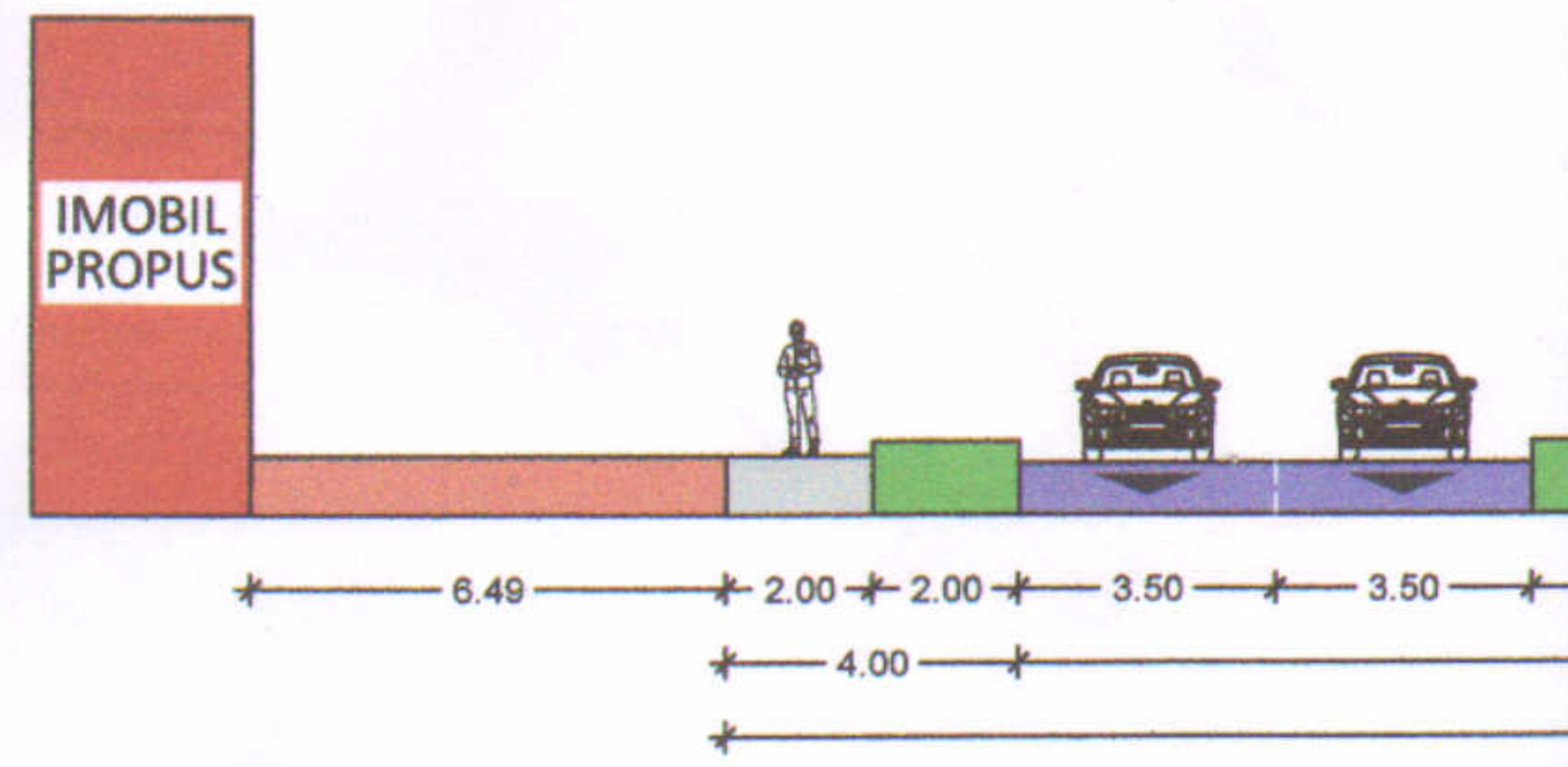
SECTIUNE S1 - S1' PROFIL STRADAL - STR. DOAMNA GHICA scara 1:200
