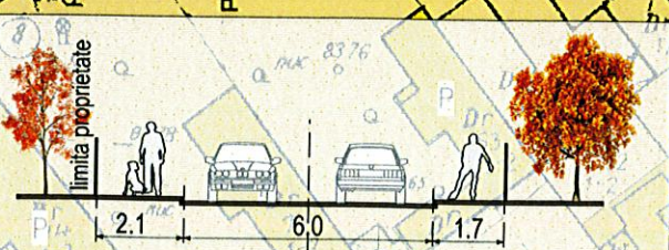
Profil A-A - str. Hispania - existent si mentinut, sc. 1:200
