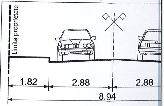
Profil stradal str. Plugusor
