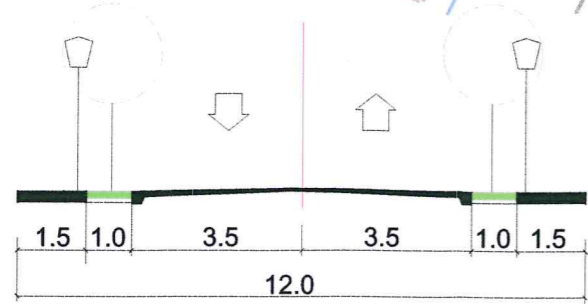
Str. Prof. Ion Ursu - Profil stradal reglementat
